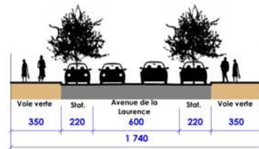
COUPE G - PRO
