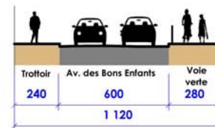
COUPE K - PRO
