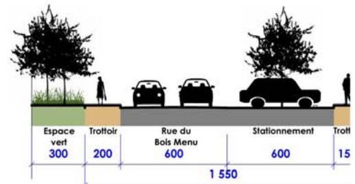
COUPE H - PRO
