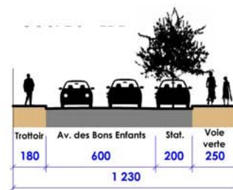
COUPE J - PRO
