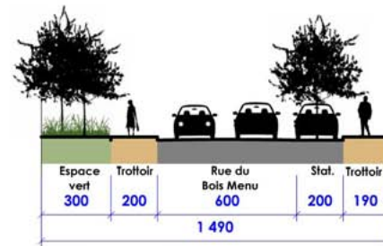
COUPE I - PRO
