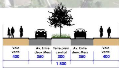
COUPE A - PRO
