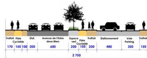
COUPE E - PRO
