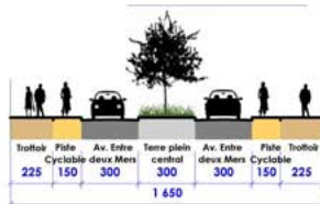
COUPE C - PRO
