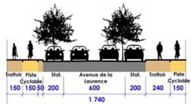
COUPE F - PRO
