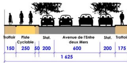
COUPE B - PRO
